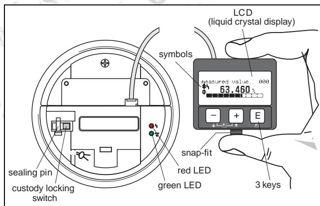
LC-Display VU331
