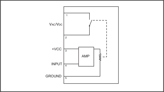
Relay Output Module
