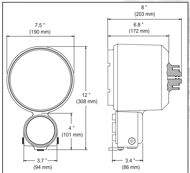
4110 HLE Dimensions
